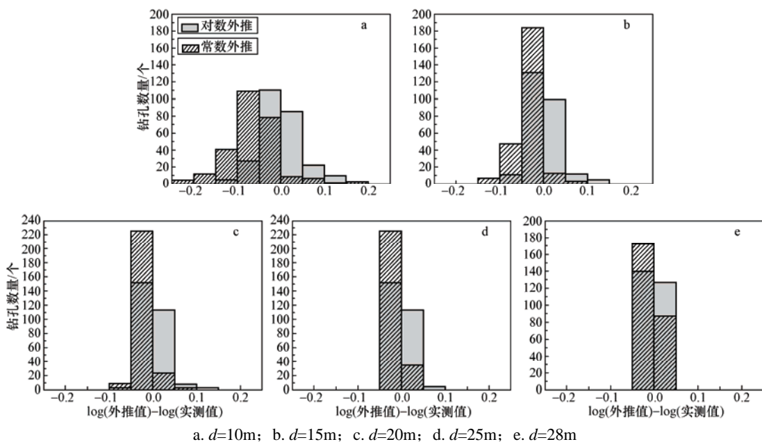
图 4 常数外推法、对数线性外推法 \bar{v}_s(30) 的残差直方对比图
