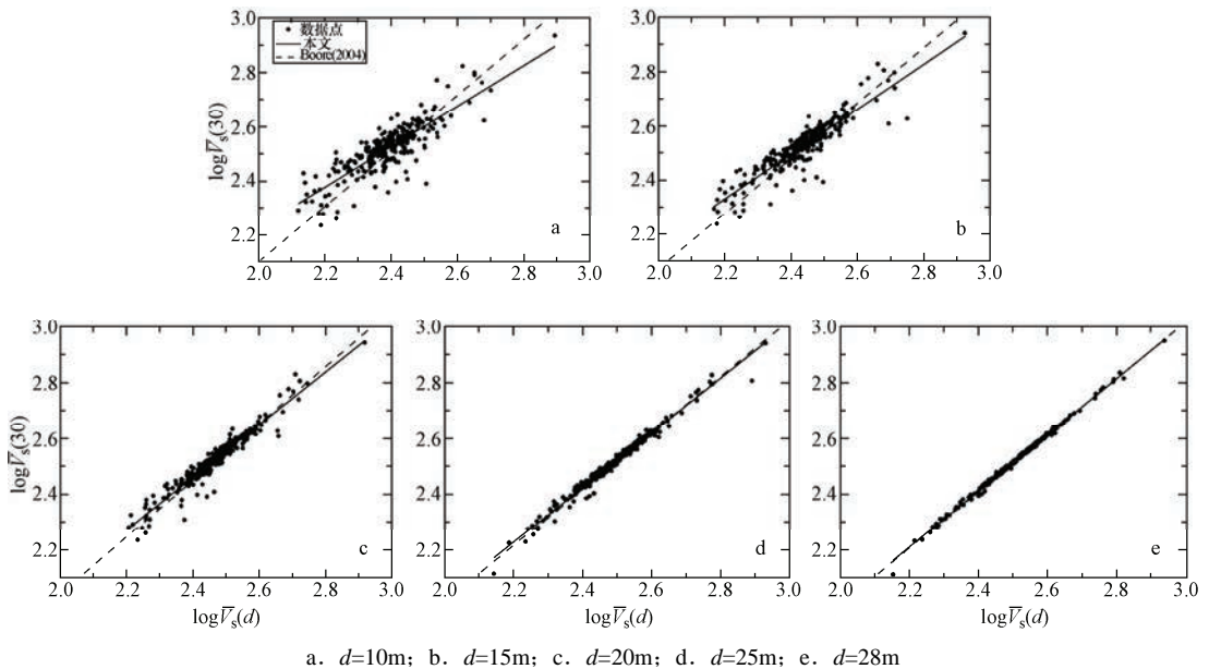
图 3 不同深度处 \bar{V}_s(d) 与 \bar{V}_s(30) 的对数线性拟合图
